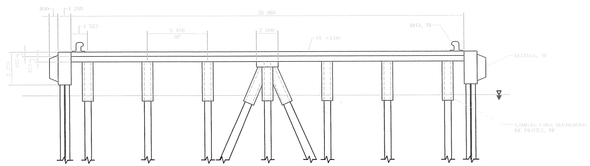
A SECCIÓN ESTRUCTURAL ESCALA: 1:100
